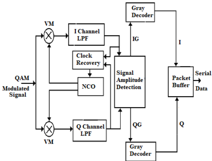
VM : VEDIC MULTIPLIER
